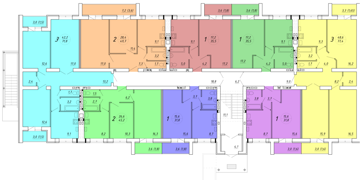
ПЛАН 1 ЭТАЖА СЕКЦИЯ 1
